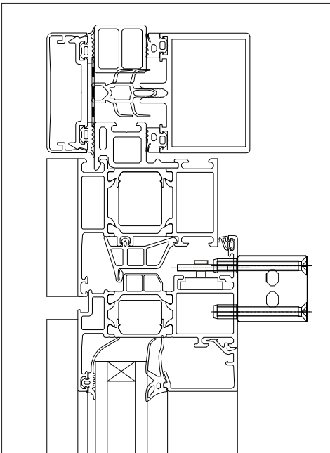
Abb. 3: Flügelmontage am Kippfenster mit Riegelantrieb KLM L
