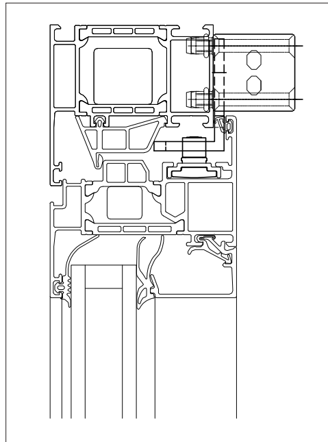
Abb. 4: Rahmenmontage am Kippfenster mit Riegelantrieb KLMF M
