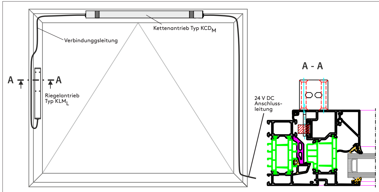
Abb. 5: Montagebeispiel am Kippflügel einwärts mit einem Kettenantrieb Typ KCD M und einem Riegelantrieb Typ KLM L
